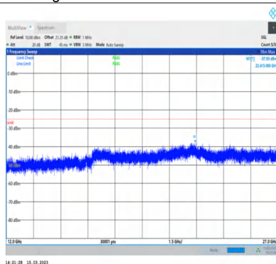
1-N7-PC3-15-20-L-1-DFT-PI2BPSK-Inner_1RB_Left- 1@1-12000-27000-Ant1-22415.00--37.93--25-PASS
