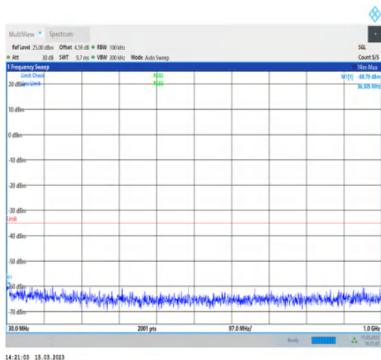
1-N7-PC3-15-20-L-1-DFT-PI2BPSK- Inner_1RB_Left-1@1-30-1000-Ant1-36.31--59.79-- 35-PASS
