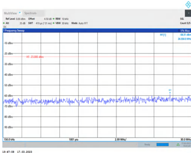
Band25-20MHz-QPSK-26140-1RB#0-Range2:0.15~30MHz
