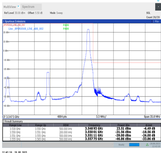
Band42_20MHz_QPSK_42990_1RB#99
