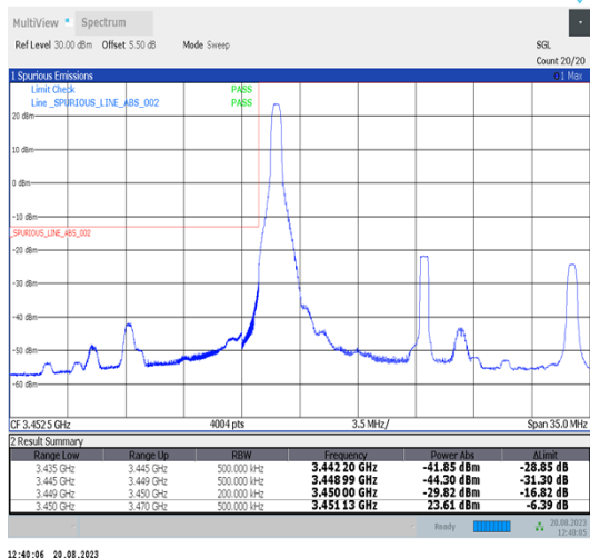
Band42_20MHz_QPSK_42190_1RB#0
