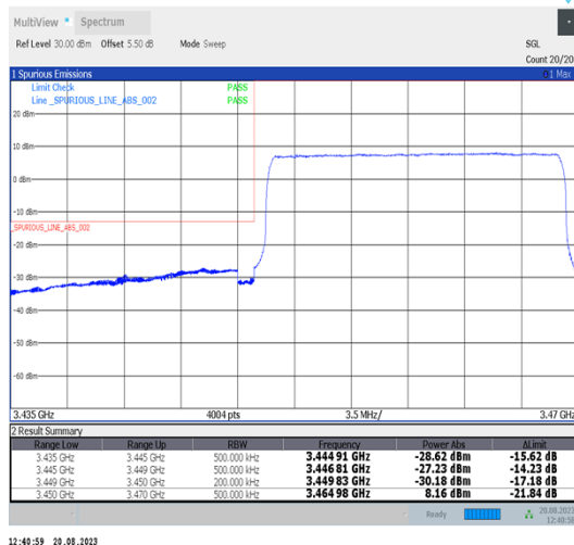
Band42_20MHz_QPSK_42190_100RB#0
