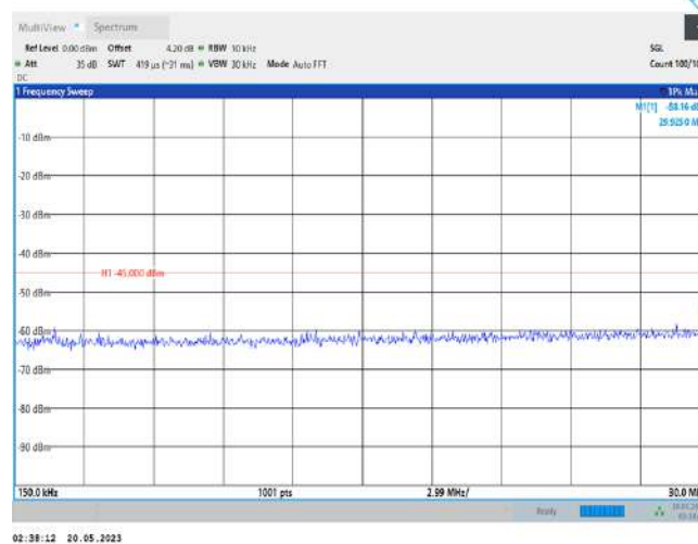
Band7-20MHz-QPSK-20850-1RB#0-Range2:0.15~30MHz
