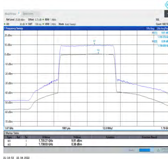
1-N66-PC3-15-40-L-2-CP-256QAM-Outer_Full-216 @0-Ant0-9.53-100%-0.00-9.53-PASS-≤13
