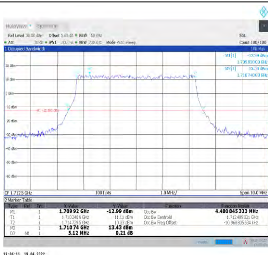
1-N66-PC3-15-5-L-1-DFT-QPSK-Outet_Full-25@0-A nt0-4.481-5.120-<5-PASS
