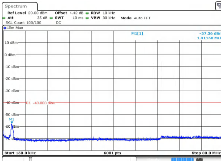
Band48-20MHz-QPSK-55340-1RB#0-Range2:0.15~30MHz
