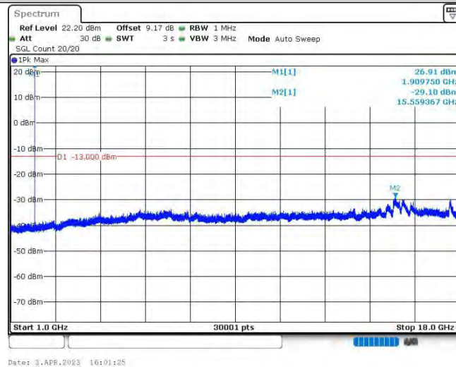
EGPRS1900-512-1000~18000MHz
