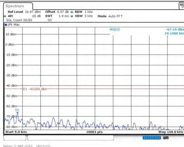
EGPRS1900-661-0.009~0.15MHz
