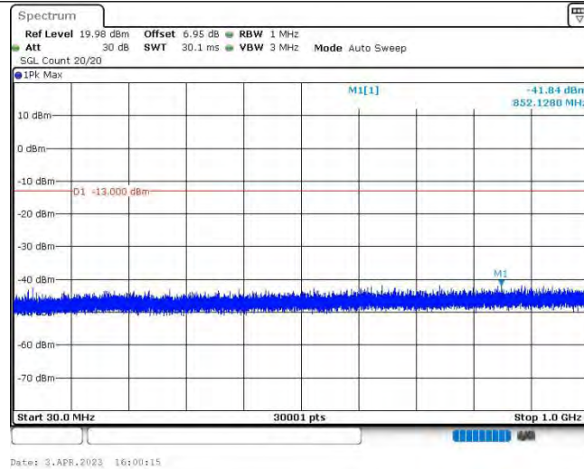
EGPRS1900-512-30~1000MHz
