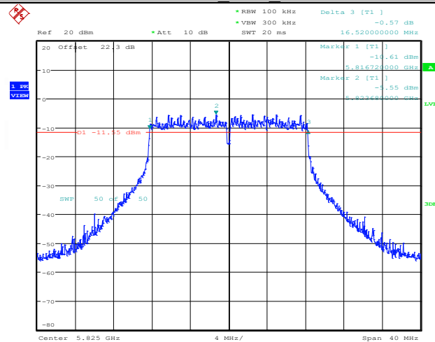
11A Ant1 5825
