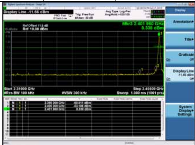
2402MHz(2.3GHz – 2.4GHz)
