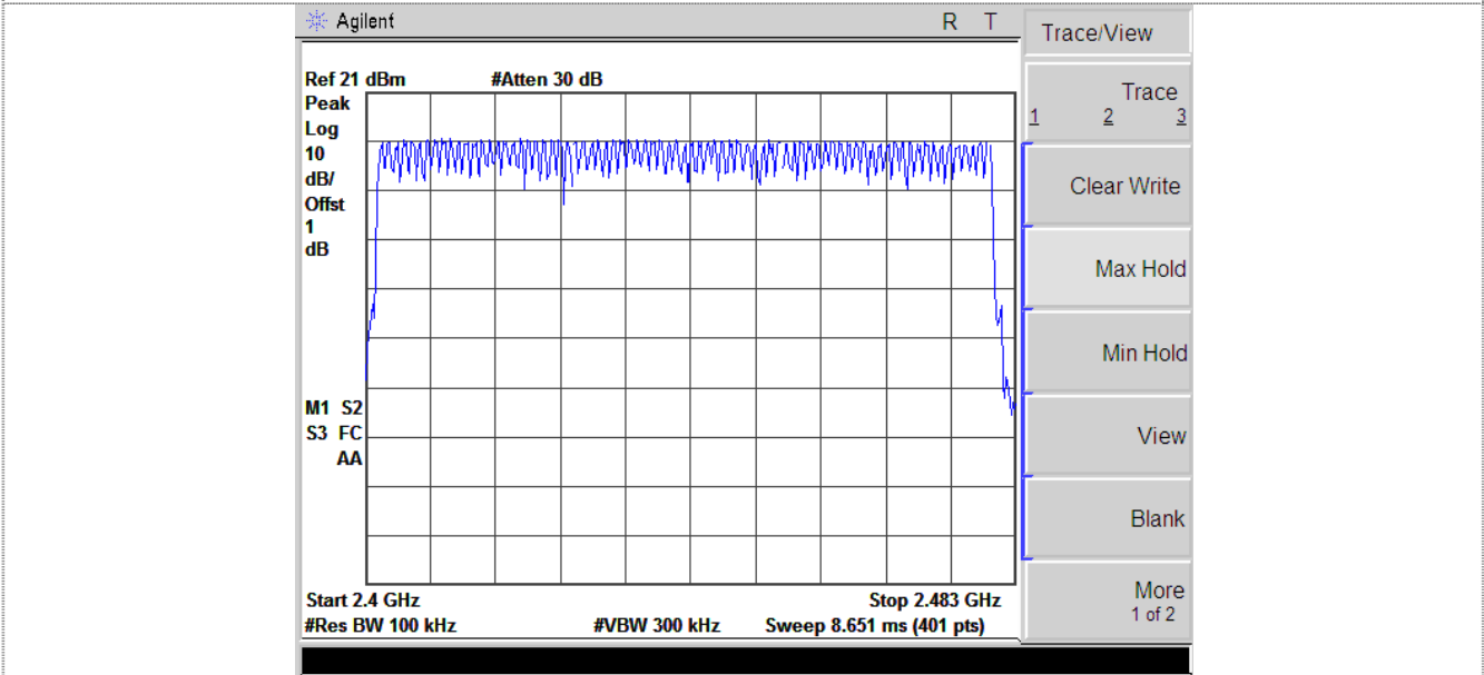
\pi/4 DQPSK
