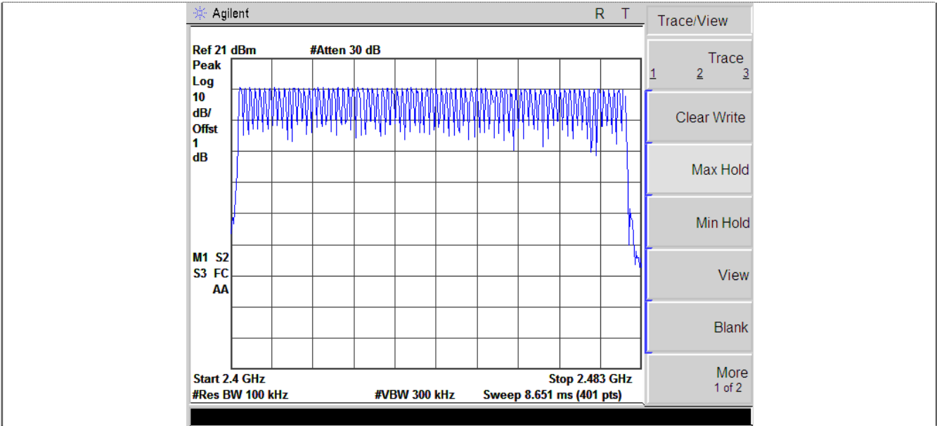
GFSK
