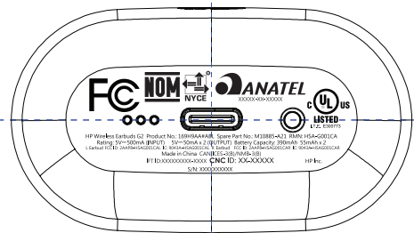
BOTTOM
