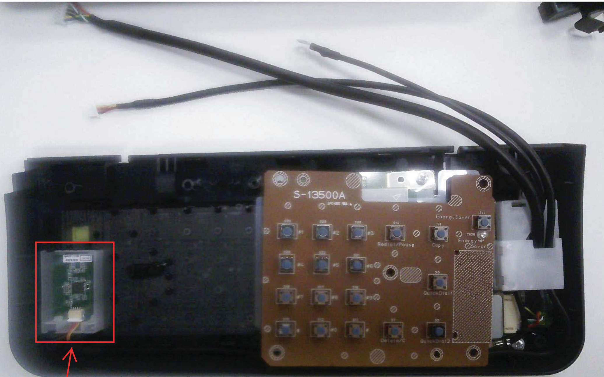
NFC Module
