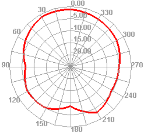
2500.000MHz E2
