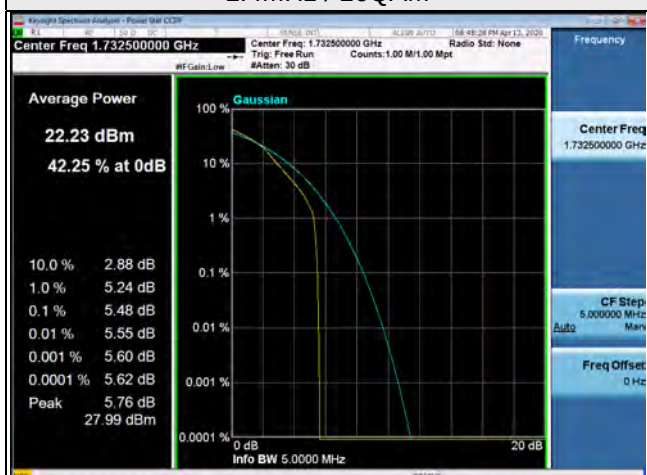
5MHz / 16QAM
