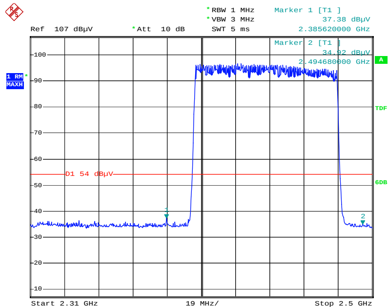
8DPSK -hopping-Ave
