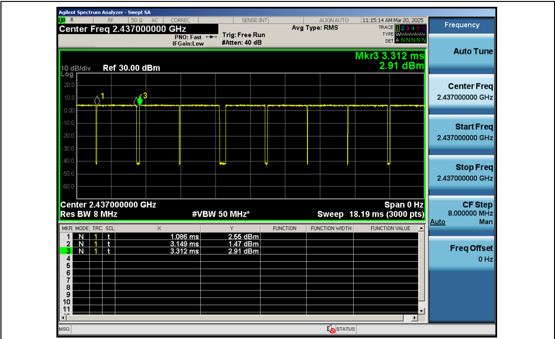
NTNV-11G-Ant1-2437
