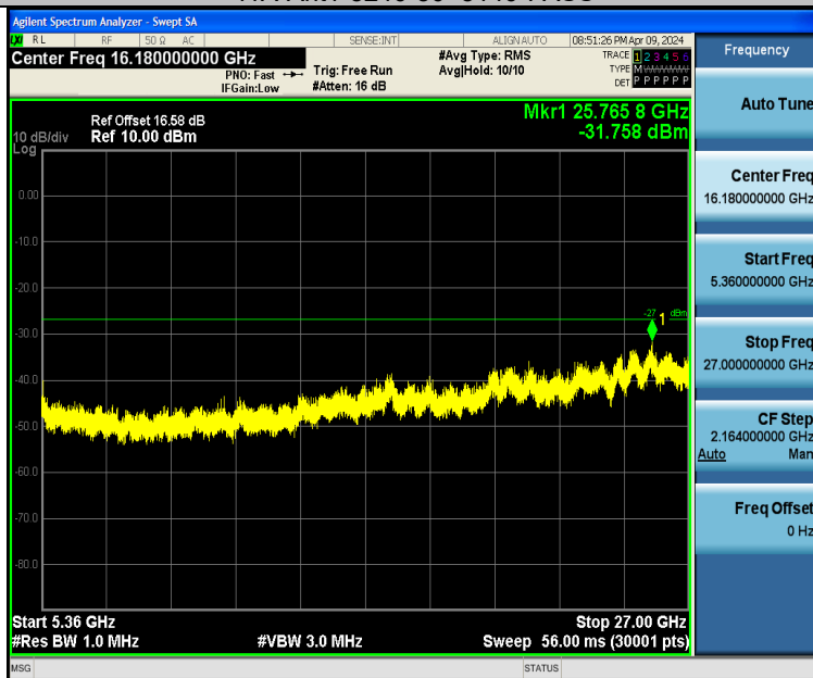
11A-Ant1-5240-5360~27000-PASS
