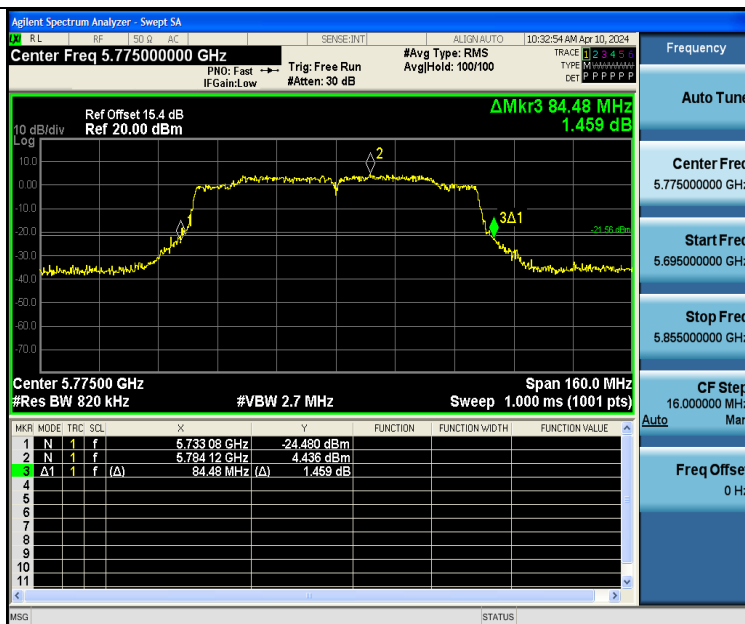
11AC80SISO-Ant1-5775
