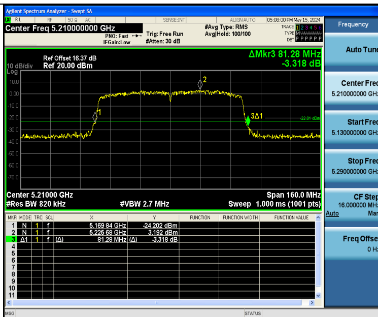
11AX80SISO-Ant1-5210
