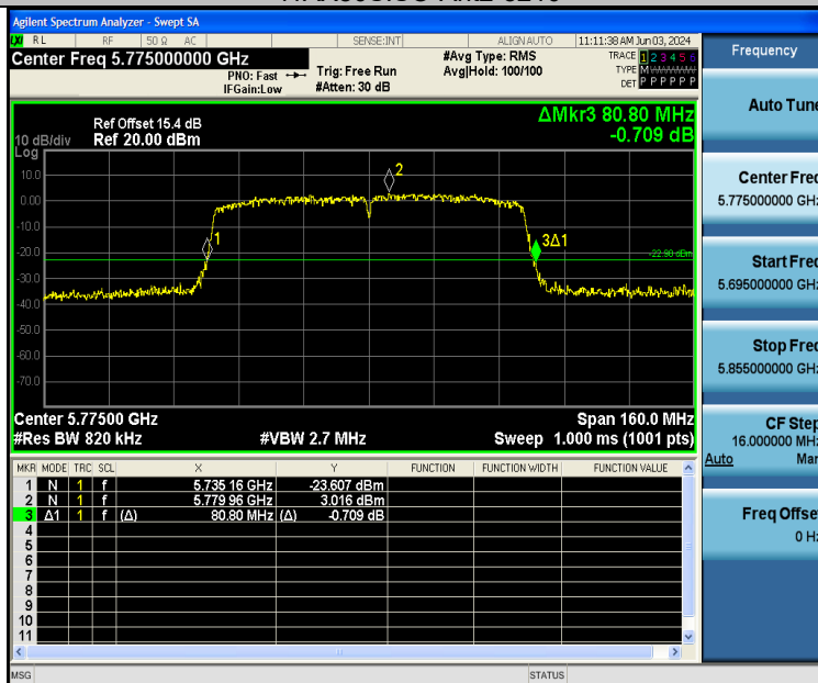
11AX80SISO-Ant2-5775
