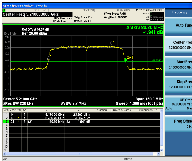
11AX80SISO-Ant2-5210
