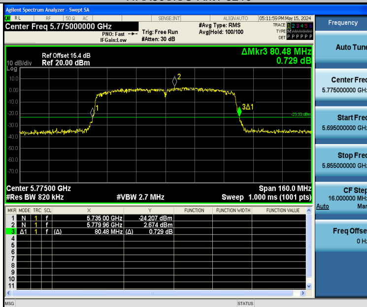
11AX80SISO-Ant1-5775
