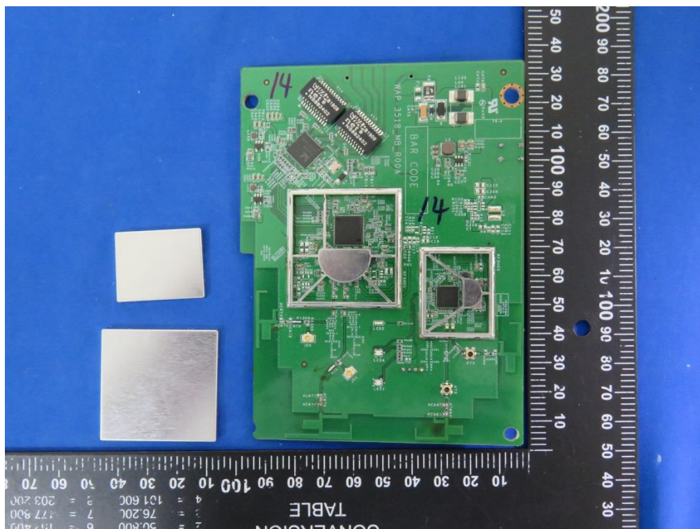
Wi-Fi 2.4G Module (Chip)
