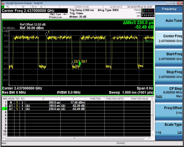
NTNV-11G-Ant1-2437
