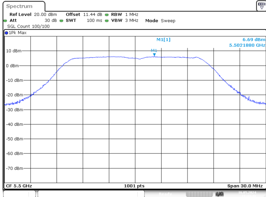
PSD NVNT a 5500MHz Ant1
