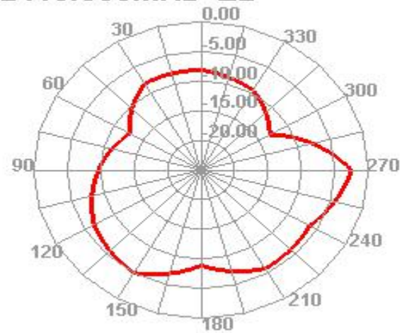
2410.000MHz E2
