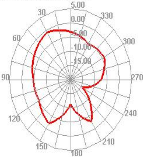
2500.000MHz E1
