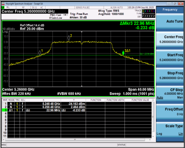
11A-Ant1-5260
