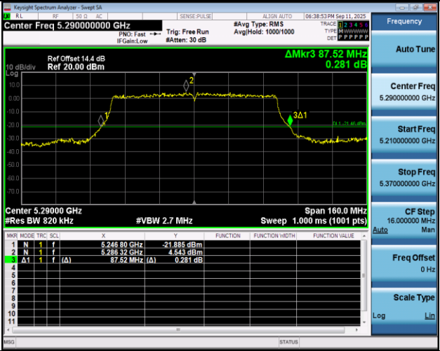
11AC80SISO-Ant1-5290
