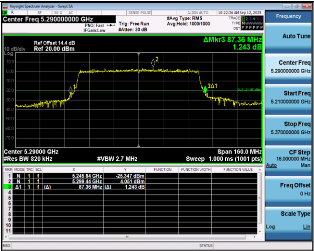
11AX80SISO-Ant1-5290
