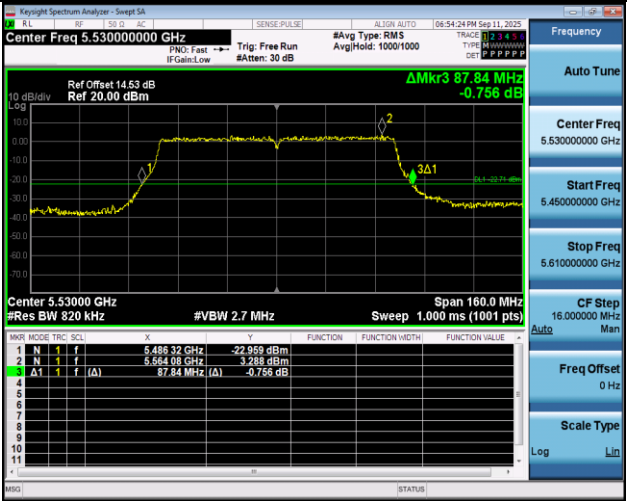
11AC80SISO-Ant1-5530
