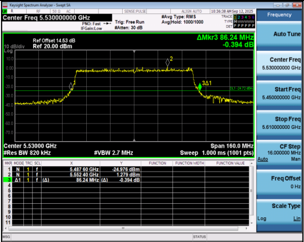
11AX80SISO-Ant1-5530
