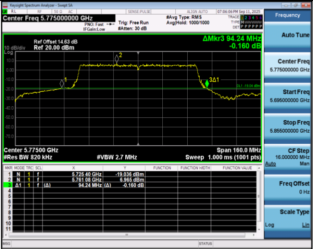
11AC80SISO-Ant1-5775
