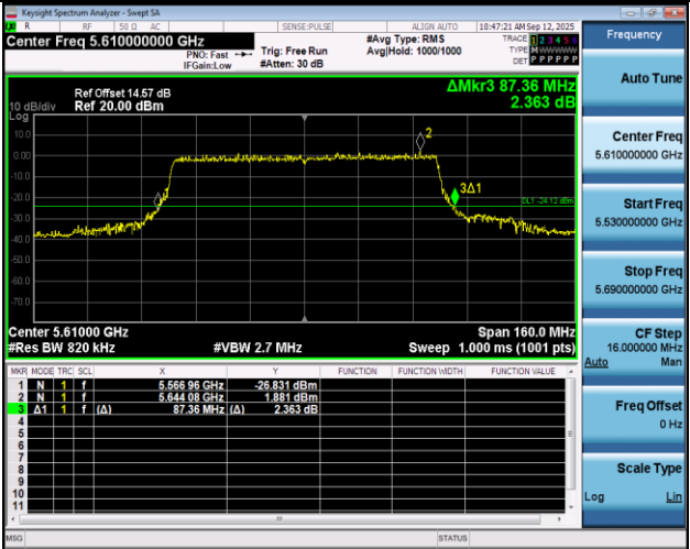
11AX80SISO-Ant1-5610
