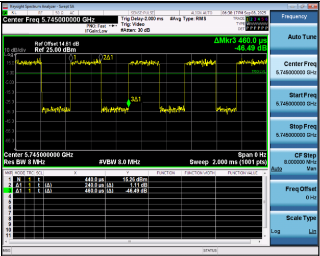
NTNV-11A-Ant1-5745
