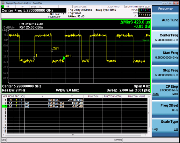
NTNV-11A-Ant1-5280
