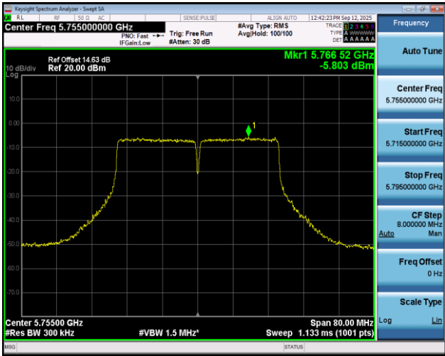
11N40SISO-Ant1-5755-PASS
