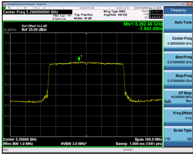
11AX80SISO-Ant1-5290-PASS
