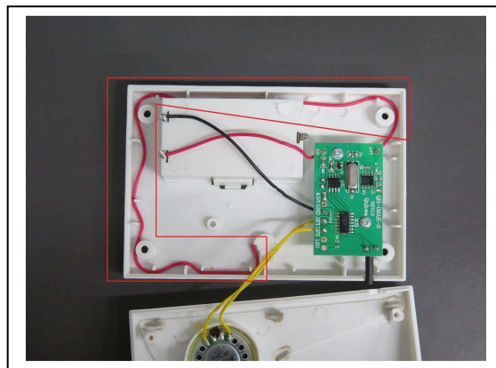
EUT Antenna
