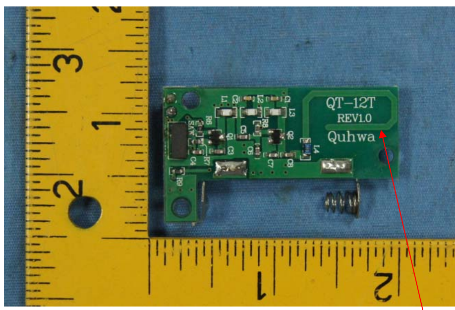
Antenna
