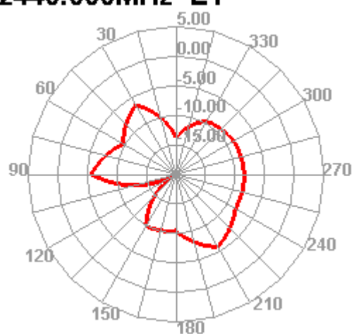
2440.000MHz E1
