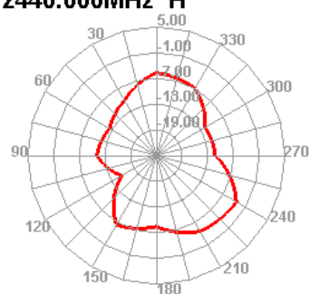
2440.000MHz H
