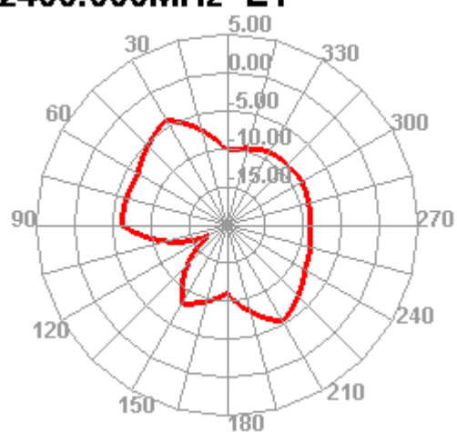
2400.000MHz E1
