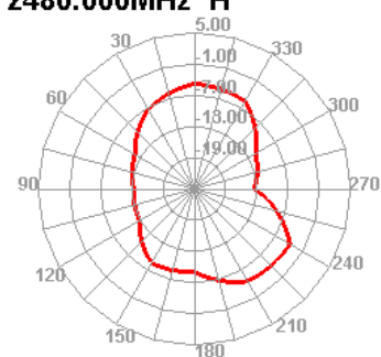
2480.000MHz H
