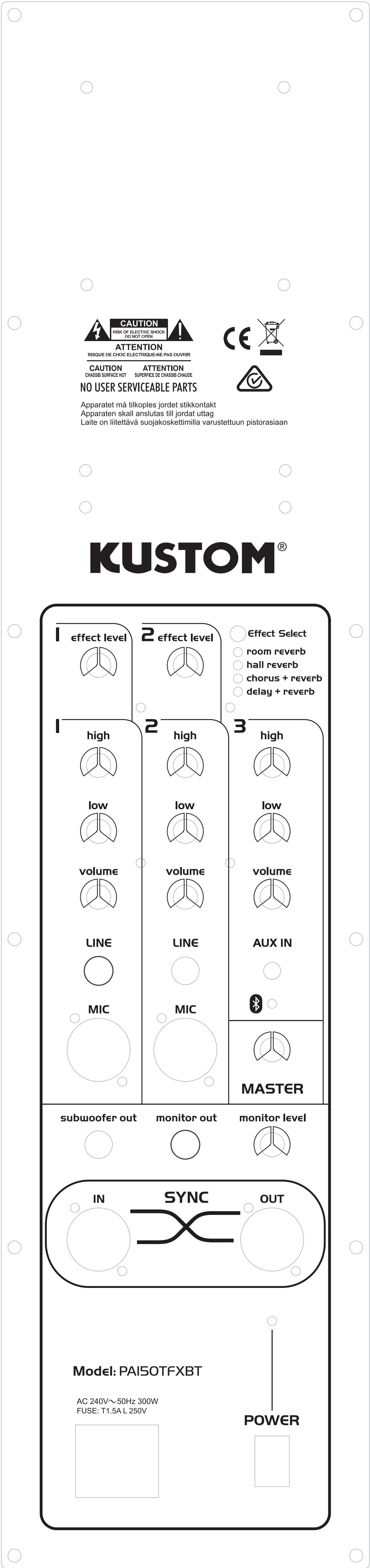
名称: PA150TFXBT输入面板丝印 丝印颜色: 白色; 底色: 黑色(喷塑)。 输入面板尺寸: 同PW150TFXBT输入面板
