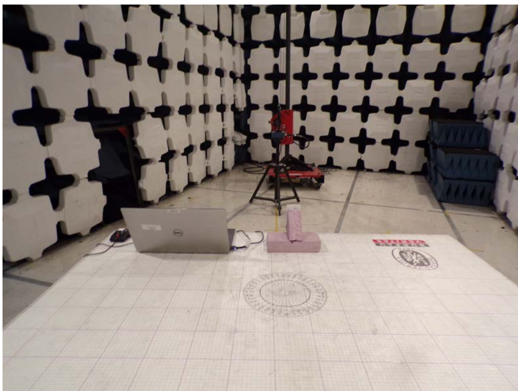
1-30MHz Perpendicular
