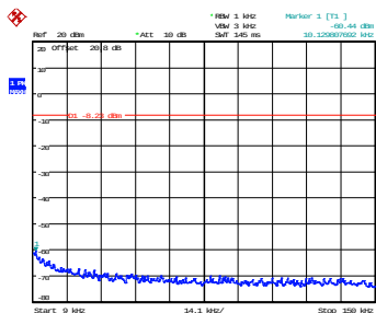
9 kHz – 150 kHz
