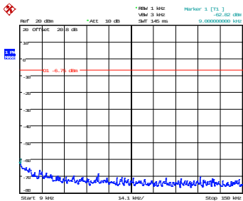
9 kHz – 150 kHz
