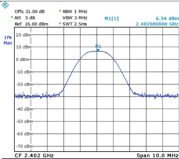
Figure 34. 2402.0 MHz, BLE
