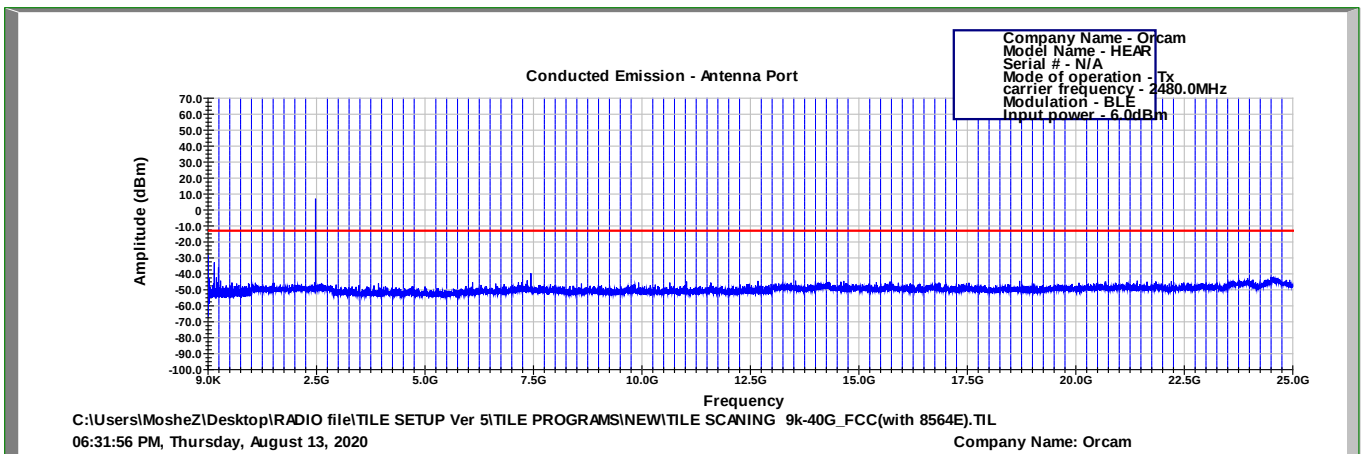
Figure 98 2480.0 MHz, BLE
