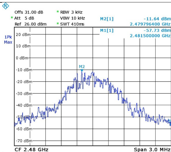
Figure 67. 2480.0 MHz, BLE
