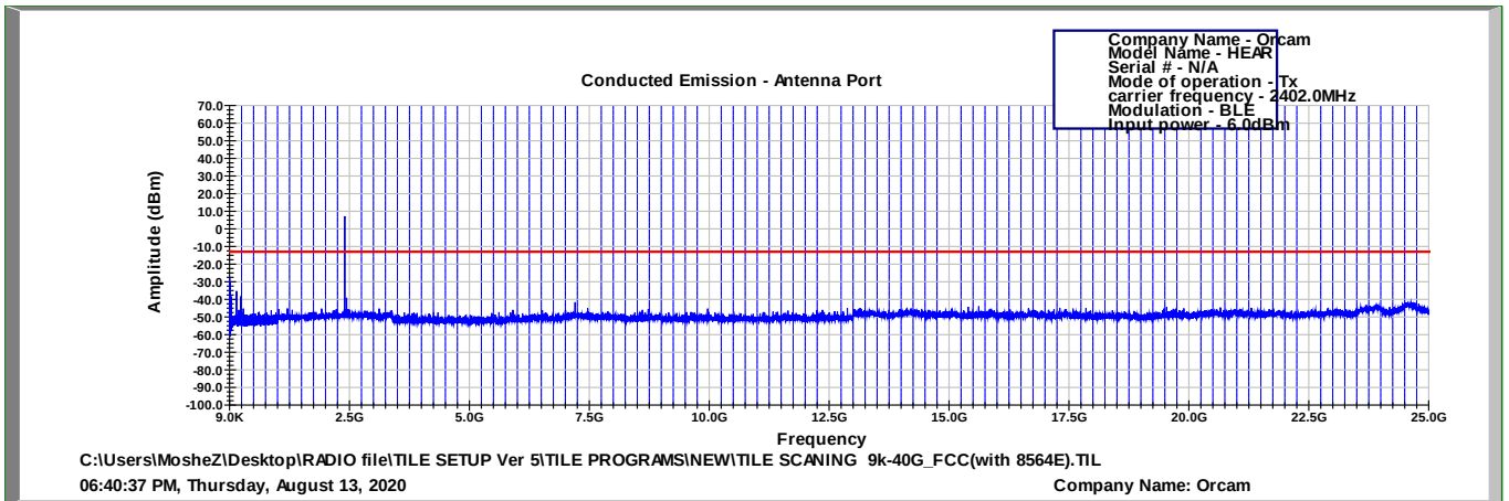
Figure 96 2402.0 MHz, BLE
