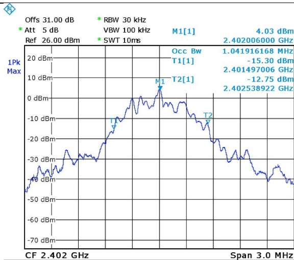
Figure 80. 2402.0 MHz, BLE
