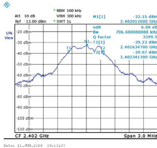
Figure 21. 2402.0 MHz, BLE
