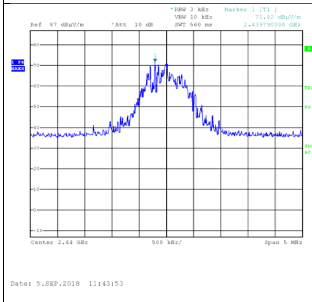
Figure 84. 2440.0 MHz, BLE
