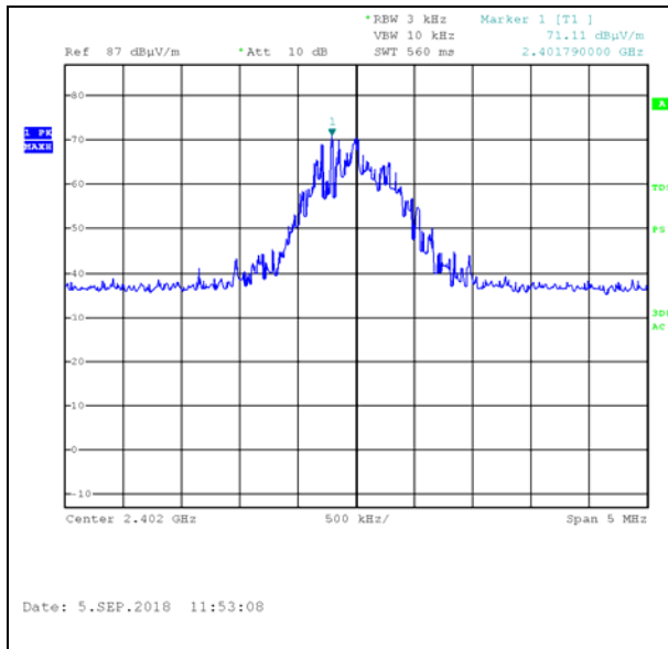
Figure 82. 2402.0 MHz, BLE
