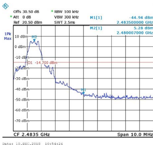
Figure 71 Band Edge High, BLE
