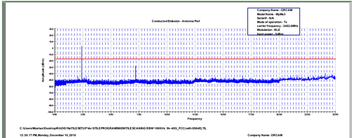
Figure 115 2402.0 MHz, BLE
