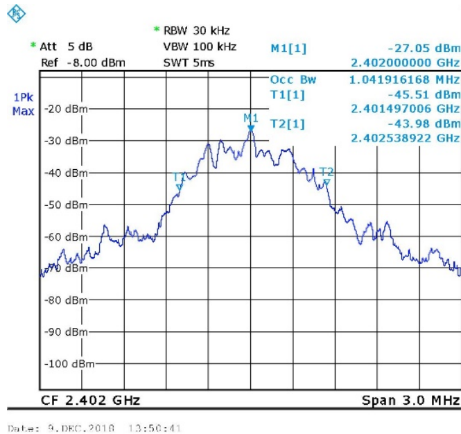
Figure 99. 2402.0 MHz, BLE
