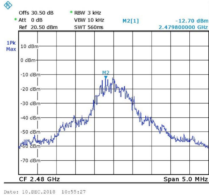
Figure 84. 2480.0 MHz, BLE
