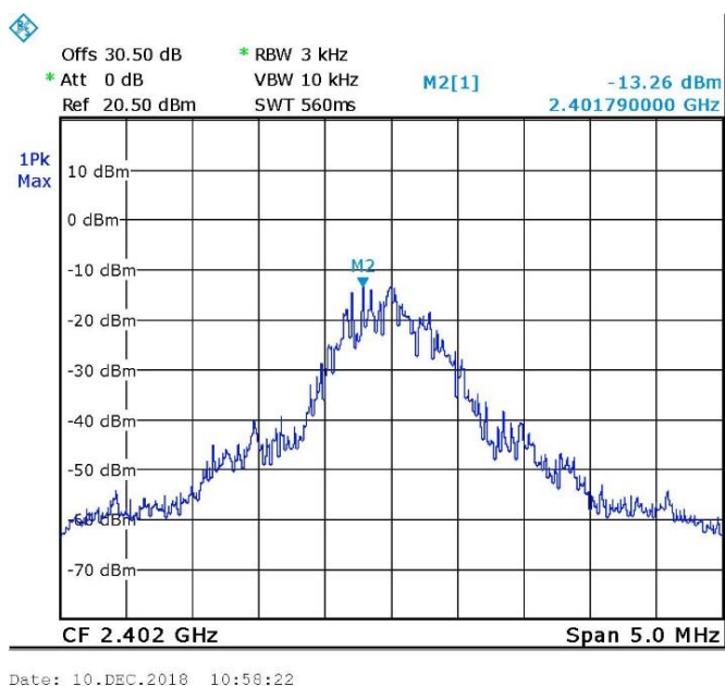
Figure 82. 2402.0 MHz, BLE
