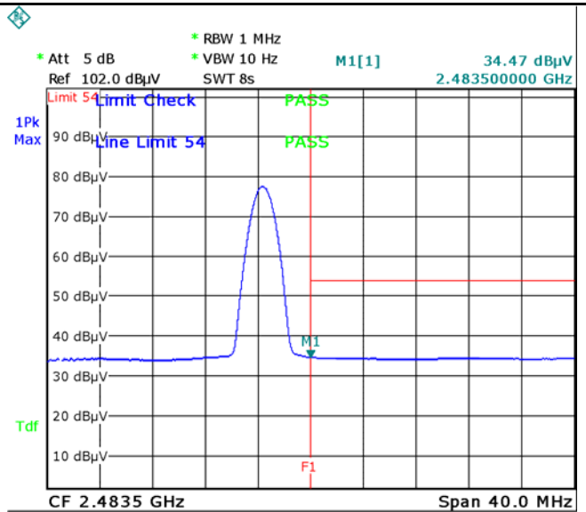
GFSK-Right Side-AV
