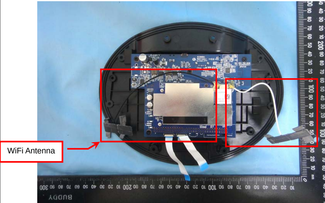
EUT Photo 7 )
