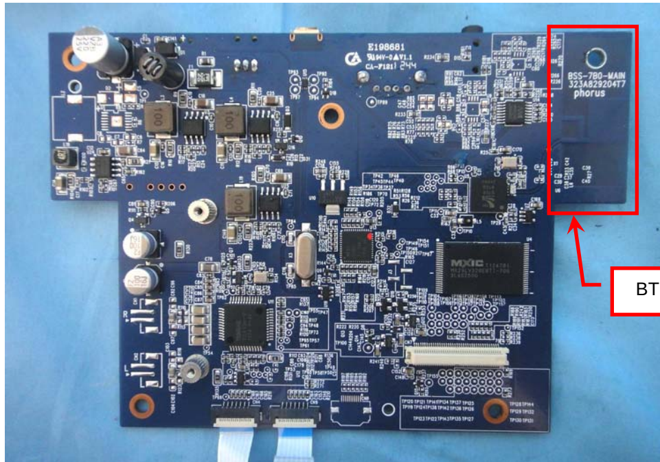
EUT Photo 9 )
