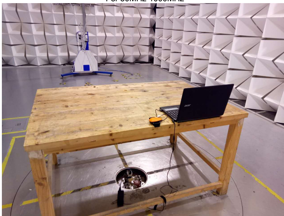
For 30MHz-1000MHz
