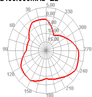
2450.000MHz E2
