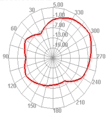
2500.000MHz H
