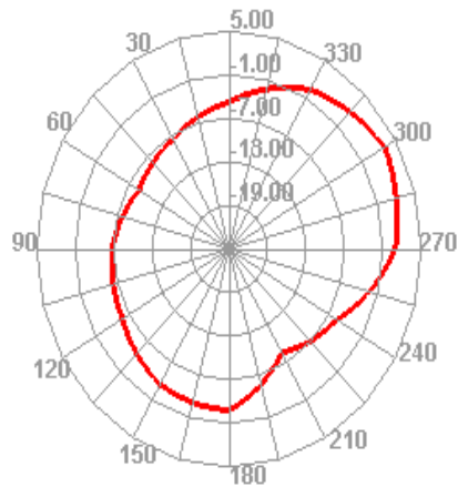
2400.000MHz H
