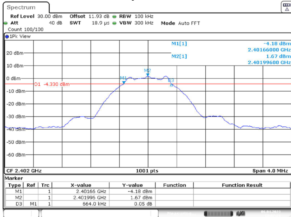
1Mbps_Ant1_2402
