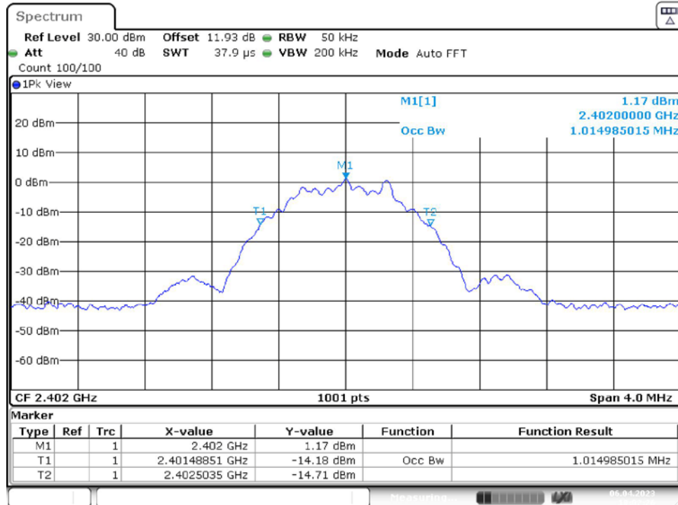
1Mbps_Ant1_2402
