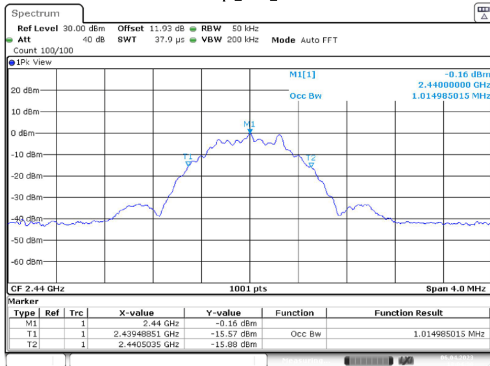
1Mbps_Ant1_2440
