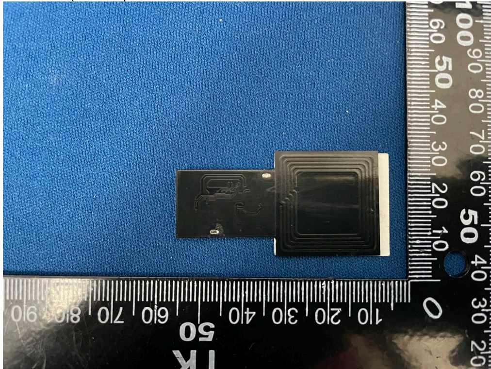
(3) EUT Photo (Antenna)
