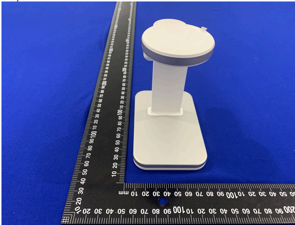
6) EUT Photo
