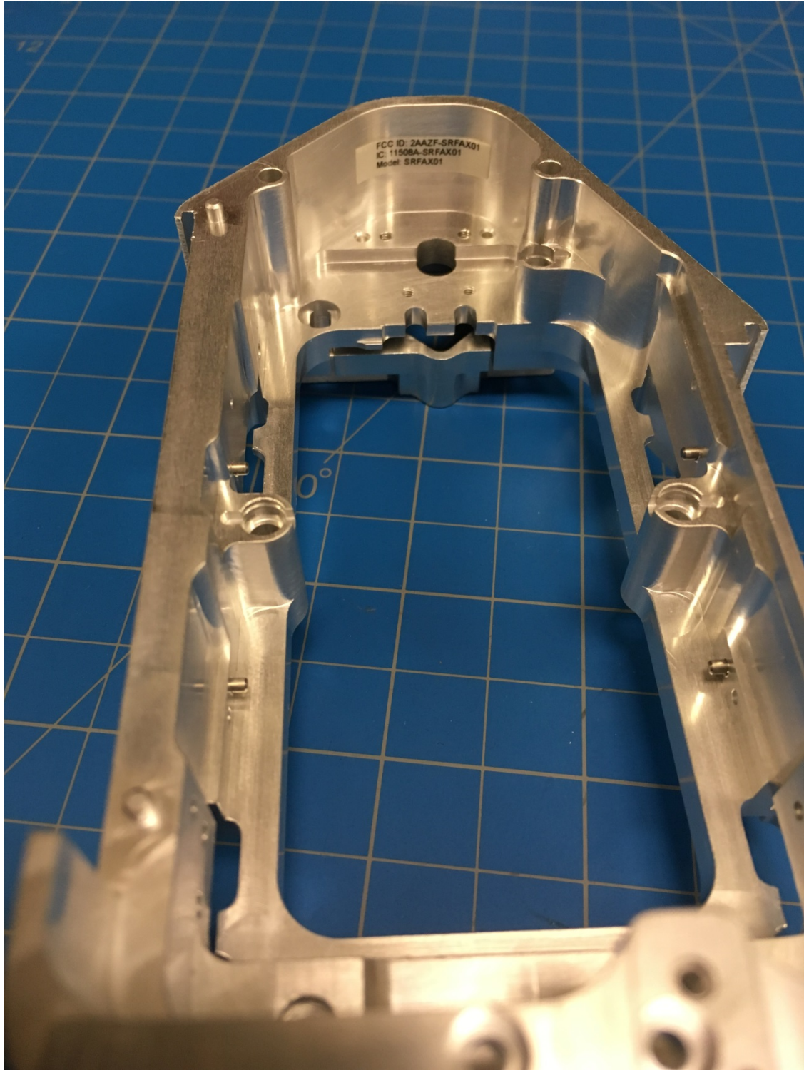
Labeled Module 01
