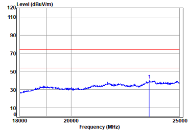
BLE_2M_TX_CH_39_Vertical
