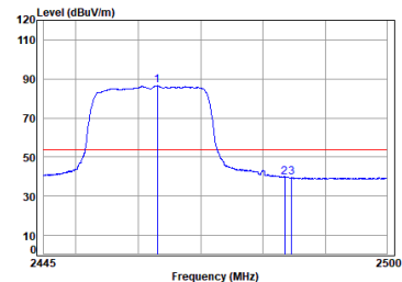
11n_HT(20M)_TX_CH_11_Vertical-Avg
