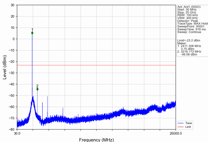
802.11b_LCH_2412MHz_Ant1 (SISO)_NTNV
