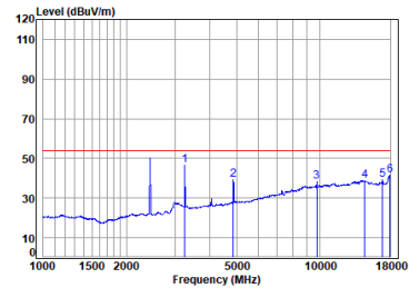
11g_TX_CH_06_Horizontal-Avg
