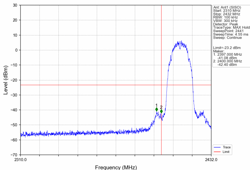
802.11b_LCH_2412MHz_Ant1 (SISO)_NTNV
