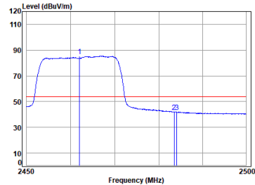
11n_HT(20M)_TX_CH_11_Vertical-Avg
