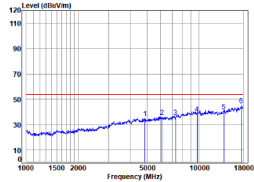
11n_HT(20M)_TX_CH_06_Horizontal-Avg
