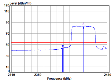
11n_HT(40M)_TX_CH_03_Vertical-Avg
