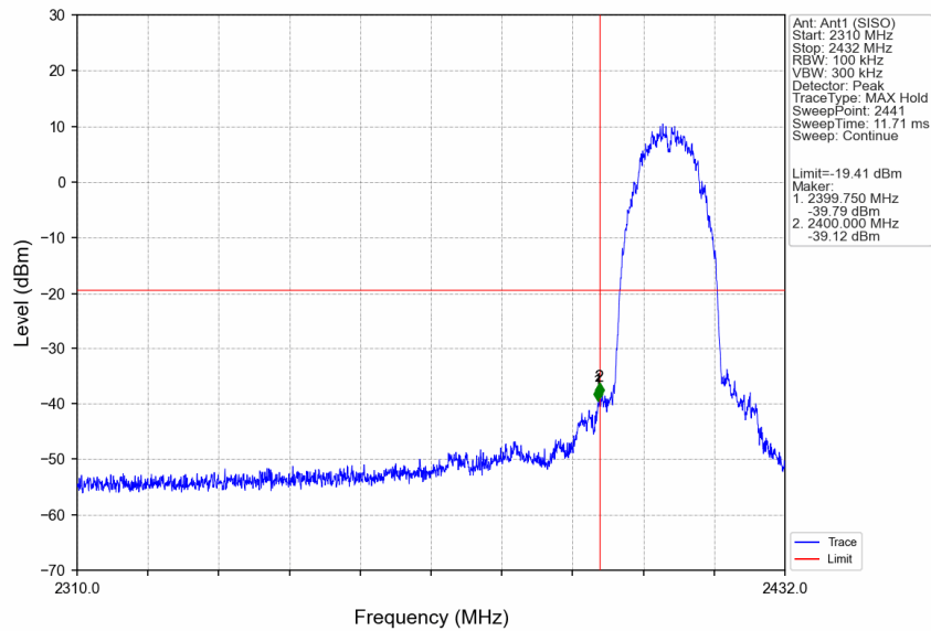
802.11b_LCH_2412MHz_Ant1 (SISO)_NTNV
