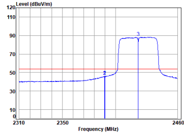
11n_HT(40M)_TX_CH_03_Horizontal-Avg
