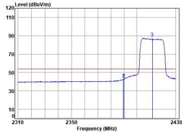
11n_HT(20M)_TX_CH_01_Vertical-Avg
