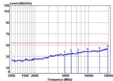
11n_HT(20M)_TX_CH_06_Vertical-Avg
