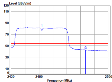
11n_HT(40M)_TX_CH_09_Vertical-Avg
