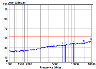
11b_TX_CH_01_Vertical-Avg
