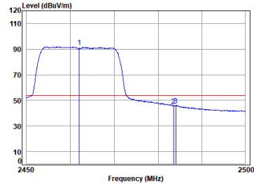
11n_HT(20M)_TX_CH_11_Horizontal-Avg
