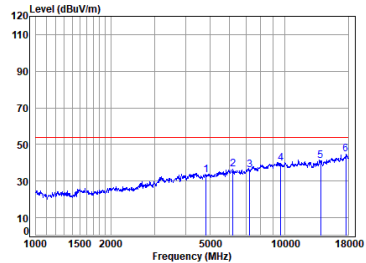
11b_TX_CH_01_Horizontal-Avg
