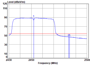
11n_HT(40M)_TX_CH_09_Horizontal-Avg
