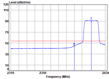
11n_HT(20M)_TX_CH_01_Horizontal-Avg
