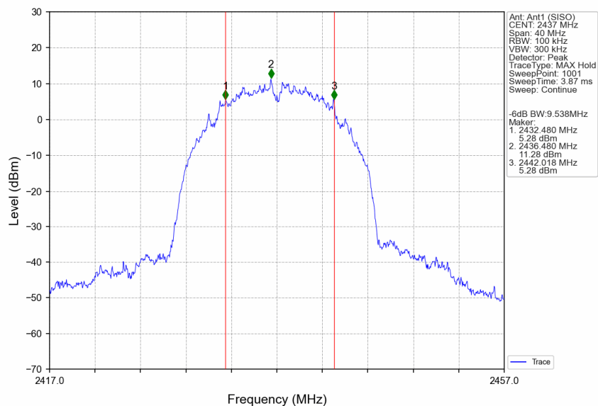
802.11b_MCH_2437MHz_Ant1 (SISO)_NTNV
